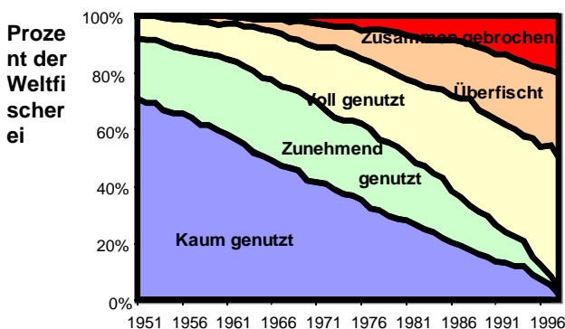
Entwicklung der globalen Fischbestände (1951-1998) © Froese/Pauly
